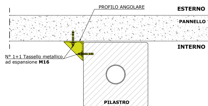
SEZIONE S1
