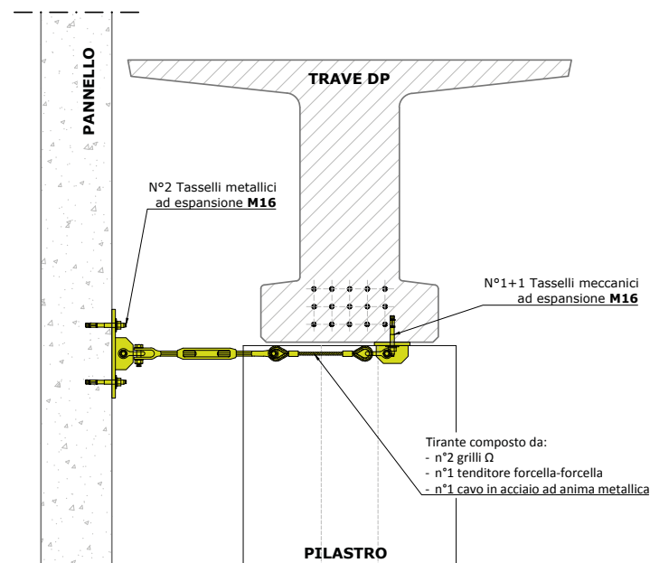
SEZIONE S1
