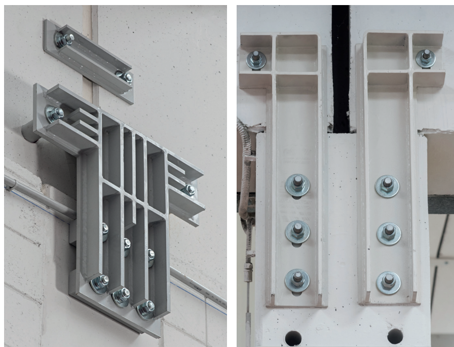
Esempi di sistemi di vincolo trave-pilastro
